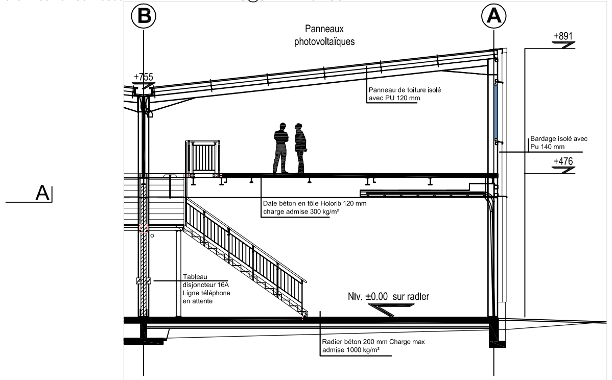
COUPE A-A
